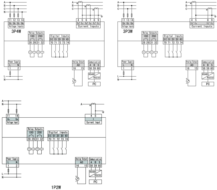
接线示意图
